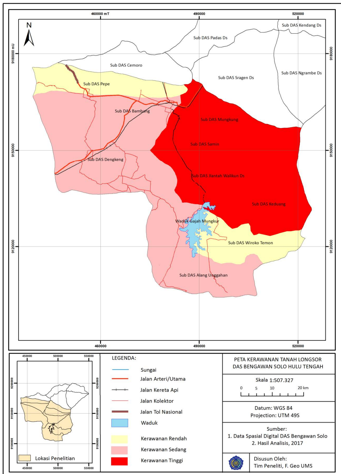
Gambar 1. Peta Kerawanan Tanah Longsor DAS Bengawan Solo Hulu Tengah
