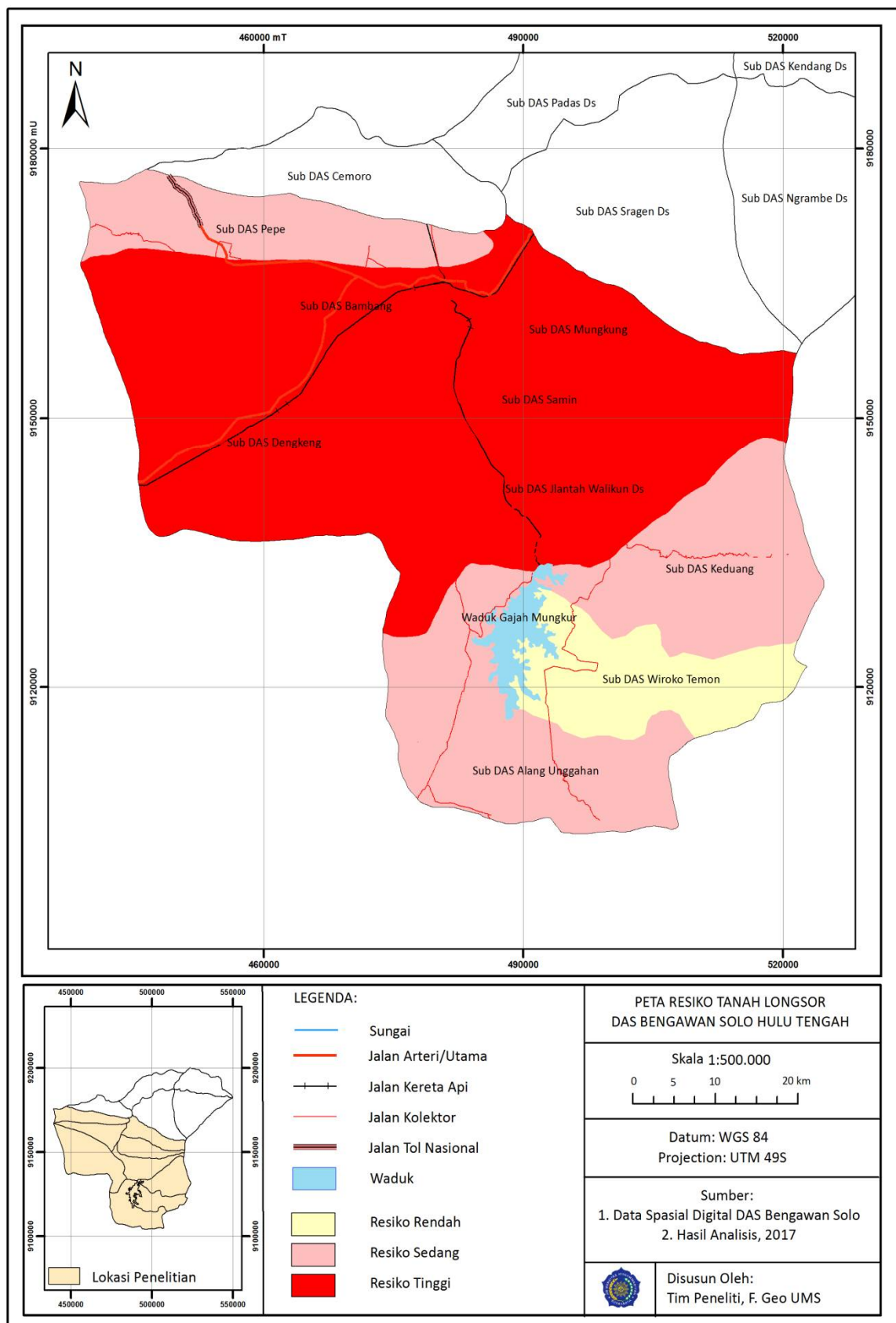
Gambar 2. Peta Resiko Tanah Longsor di DAS Bengawan Solo Hulu Tengah
