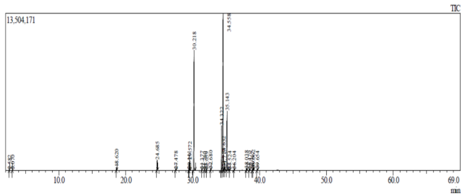
Gambar 2. Kromatogram lemak anjing hasil analisis GCMS QP 2010
