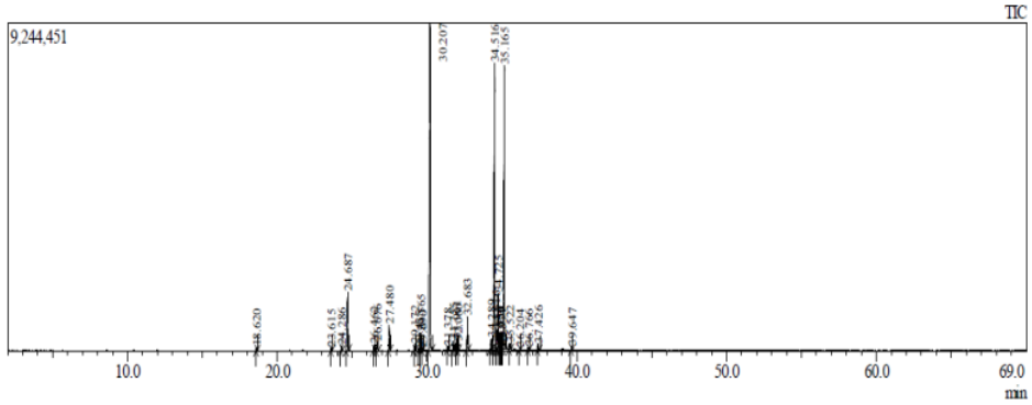
Gambar 1. Kromatogram lemak sapi hasil analisis GCMS QP 2010
